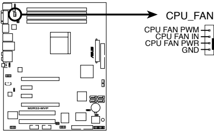
M2R32-MVP CPU fan connector
