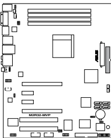
M2R32-MVP IDE connector
