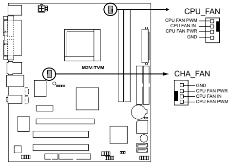
M2V-TVM Fan connectors
