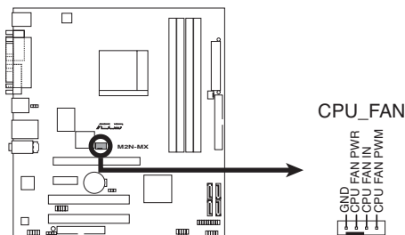
Connecteurs de ventilation de la M2N-MX
