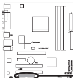
Connecteur lecteur de disquettes de la M2N-MX
