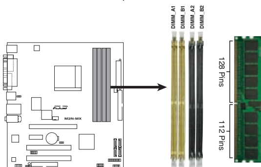
Sockets DIMM DDR2 de la M2N-MX
