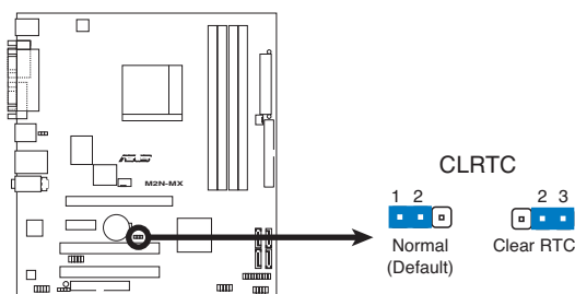
Clear RTC RAM de la M2N-MX
