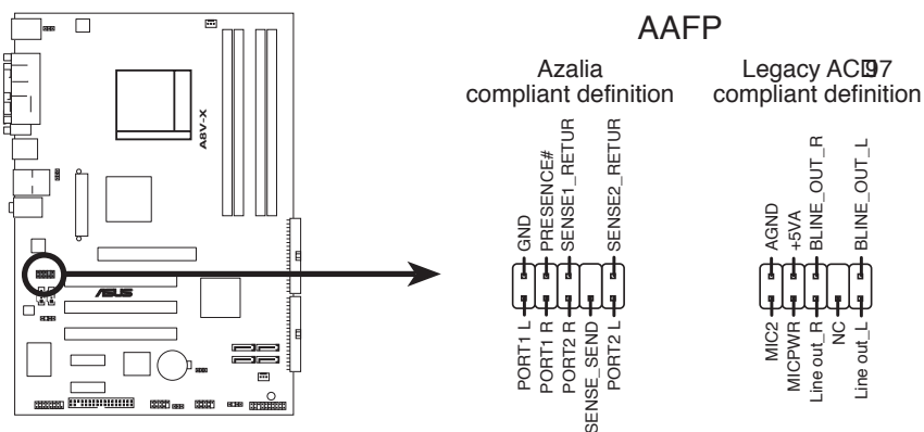
Connecteur Front panel audio de l'A8V-X
