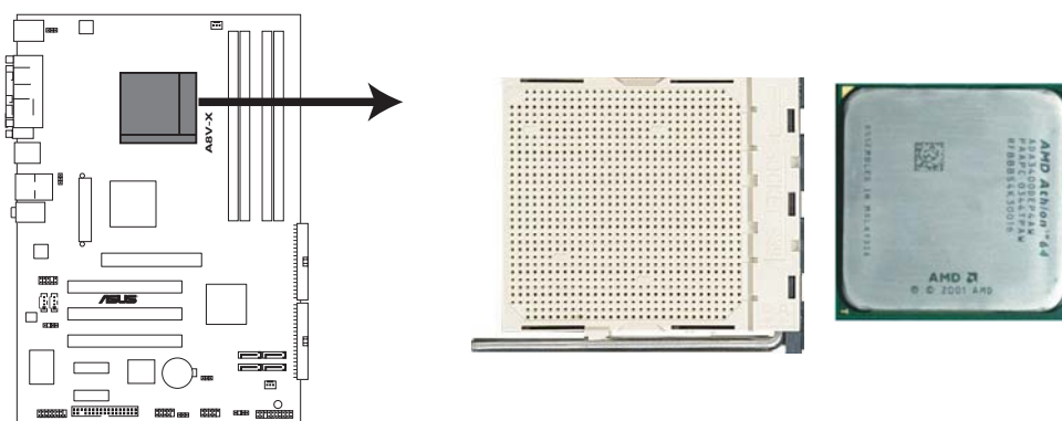
Socket 939 de l'A8V-X
