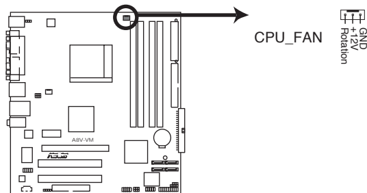
A8V-VM CPU Fan Connector
