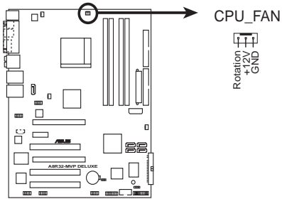
A8R32-MVP DELUXE CPU fan connector
