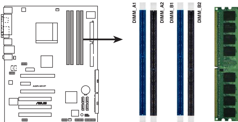
Sockets 184 broches DIMM DDR de l'A8R-MVP
