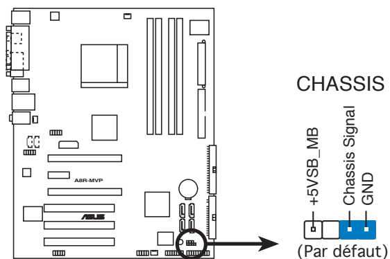
Connecteur Châssis intrusion de l'A8R-MVP
