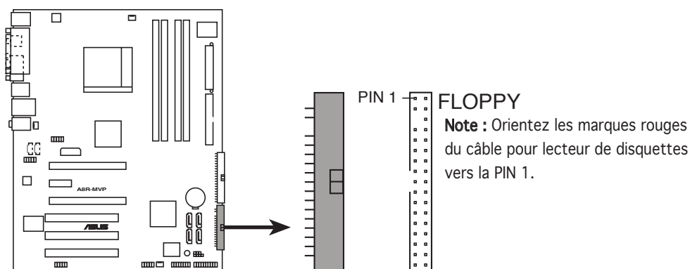
Connecteur lecteur de disquettes de l'A8R-MVP
