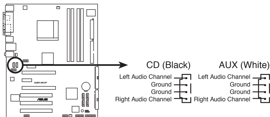
Connecteurs audio internes de l'A8R-MVP
