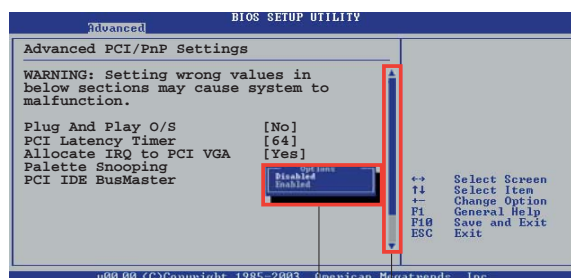
Fenêtre pop-up
