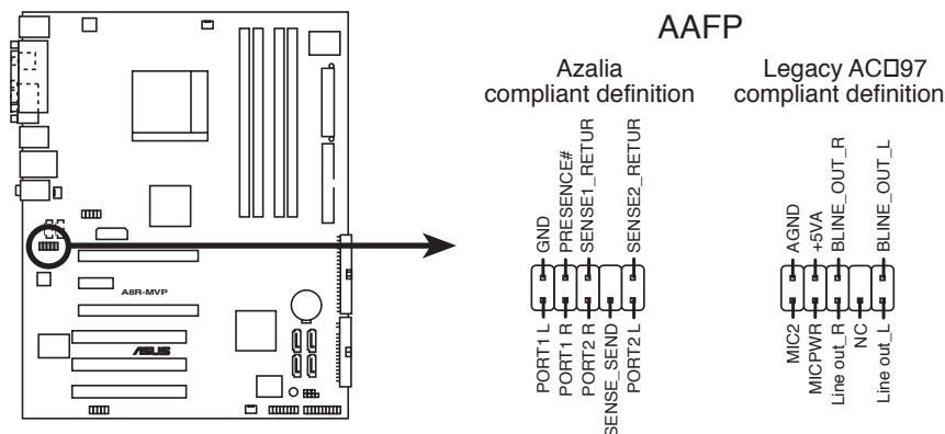
Connecteur Front panel audio de l'A8R-MVP
