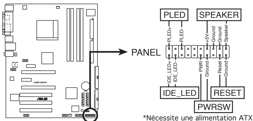
Connecteur System Panel de l'A8R-MVP
