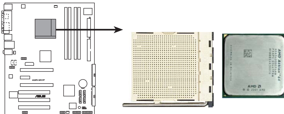
Socket 939 de l'A8R-MVP
