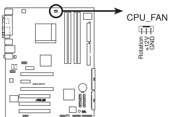
Connecteur du ventilateur CPU de l'A8R-MVP
