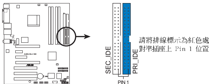
A8N-SLI SE IDE Connectors
