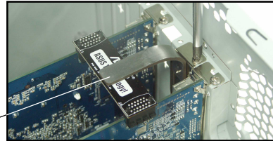
Halteblech
