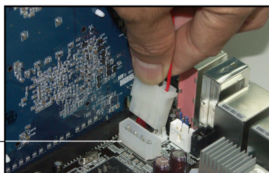
Разъем ASUS EZ Plug™
