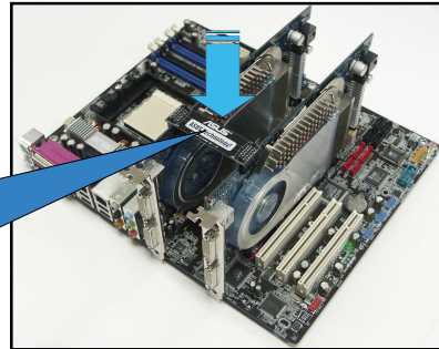
Connettore SLI
