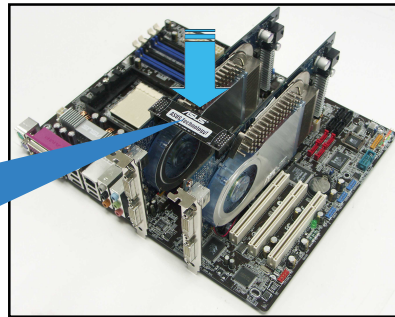
Connecteur SLI
