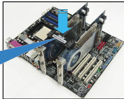
SLI-Verbindungsplatine
