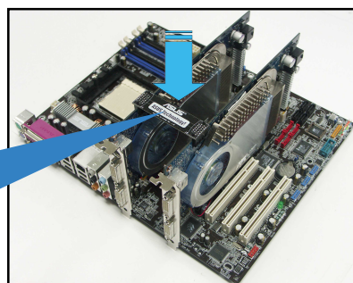
Соединитель SLI
