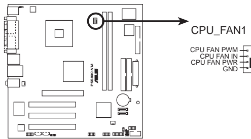
P5S800-VM CPU FAN connector
