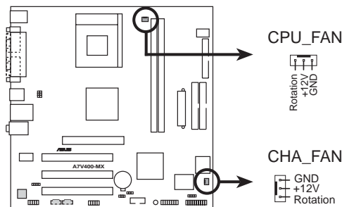
A7V400-MX 12-Volt Fan Connectors
