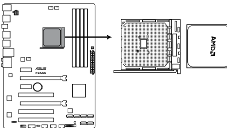
F2A55 CPU socket FM2
