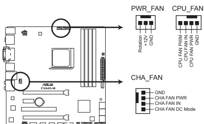
Connecteurs de ventilation de la F2A85-M
