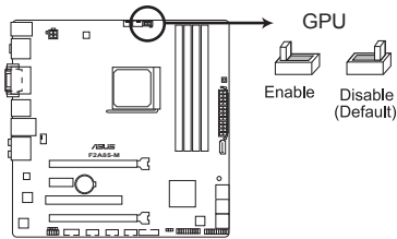
Interrupteur GPU Boost de la F2A85-M
