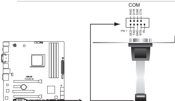
Connecteur pour port COM de la F2A85-M
