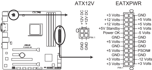
Connecteurs ATX de la F2A85-M
