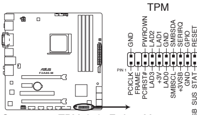
Connecteur TPM de la F2A85-M
