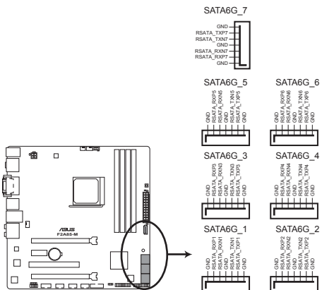
Connecteurs SATA de la F2A85-M
