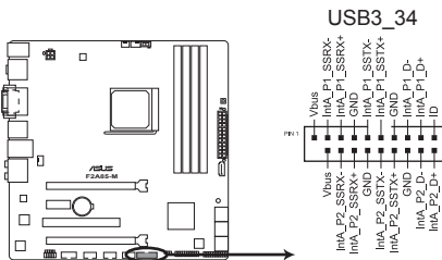
Connecteur USB 3.0 de la F2A85-M
