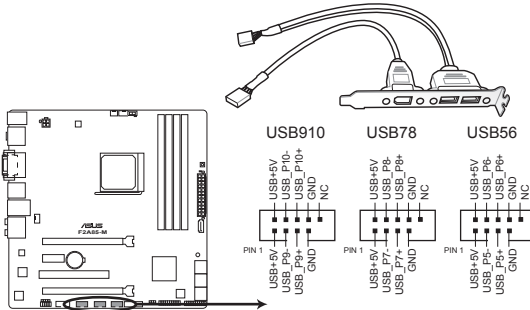
Connecteurs USB 2.0/1.1 de la F2A85-M
