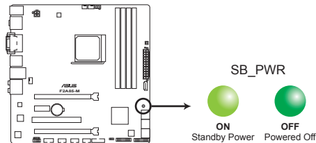
Voyant d'alimentation de la F2A85-M
