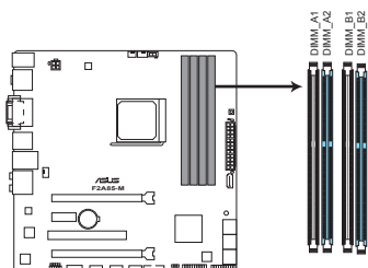
Sockets DIMM DDR3 de la F2A85-M
