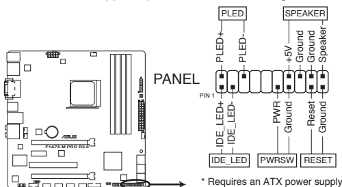
Connecteur système de la F2A85-M
