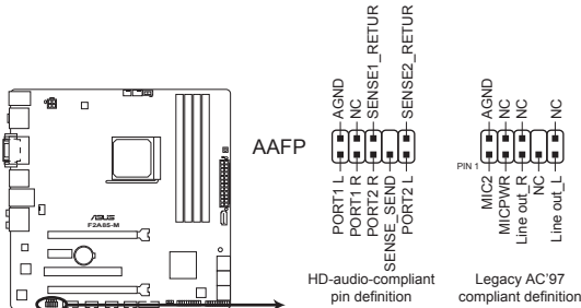
Connecteur pour port audio en façade de la F2A85-M
