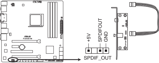
Connecteur audio numérique de la F2A85-M
