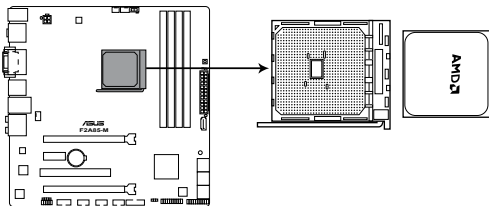
F2A85-M CPU socket FM2
