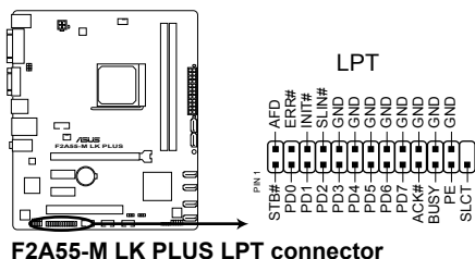
F2A55-M LK PLUS LPT connector
