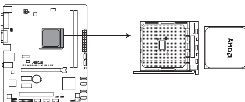
Socket de l'APU de la F2A55-M LK PLUS
