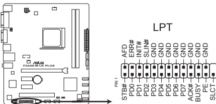
Connecteur LPT de la F2A55-M LK PLUS
