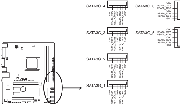
Connecteurs SATA de la F2A55-M LK PLUS
