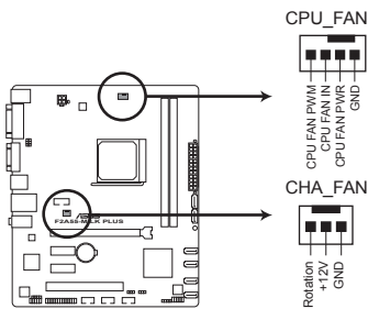
Connecteurs de ventilation de la F2A55-M LK PLUS
