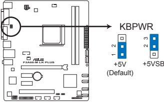
Jumper de mise en route via clavier de la F2A55-M LK PLUS
