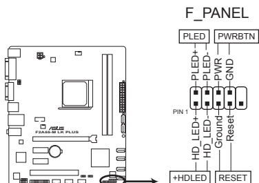
Connecteur système de la F2A55-M LK PLUS
