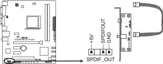
Connecteur audio numérique de la F2A55-M LK PLUS
