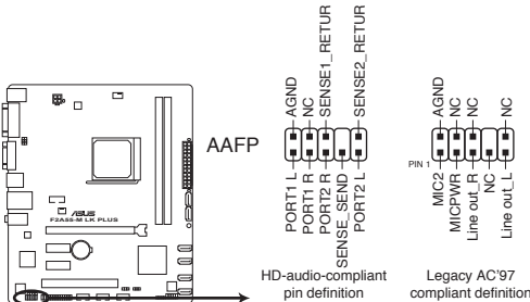
Connecteur pour port audio en façade de la F2A55-M LK PLUS
