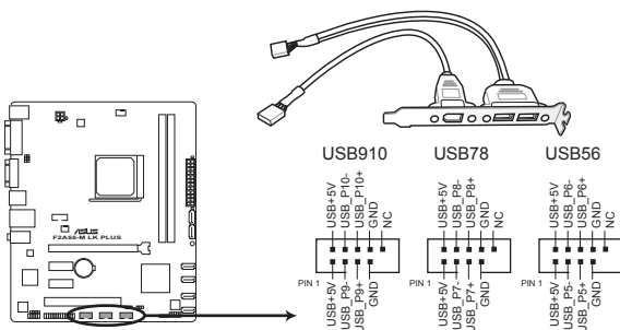
Connecteurs USB 2.0 de la F2A55-M LK PLUS
