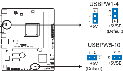
Jumper de mise en route via USB de la F2A55-M LK PLUS
