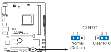
Jumper d'effacement de la mémoire RTC de la F2A55-M LK PLUS
