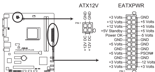
Connecteurs ATX de la F2A55-M LK PLUS
