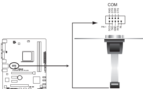
Connecteur pour port COM de la F2A55-M LK PLUS
