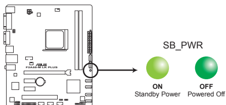
Voyant d'alimentation de la F2A55-M LK PLUS
