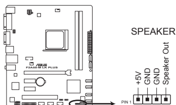
Connecteur haut-parleur système de la F2A55-M LK PLUS
