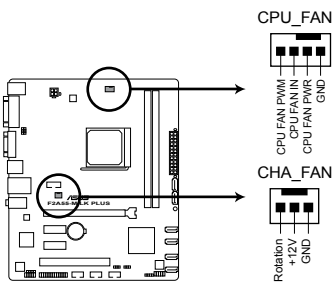
F2A55-M LK PLUS Fan connectors
