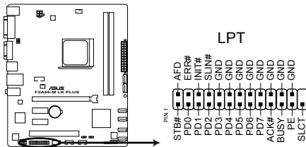
F2A55-M LK PLUS LPT connector
