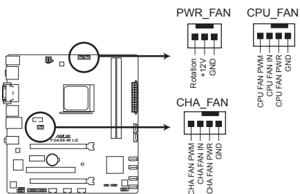
Connecteurs de ventilation de la F2A55-M LE
