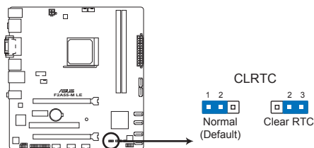
Jumper d'effacement de la mémoire RTC de la F2A55-M LE
