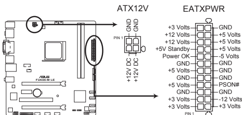
Connecteurs ATX de la F2A55-M LE
