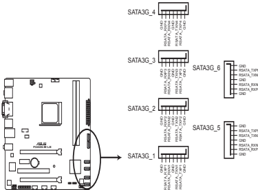
Connecteurs SATA de la F2A55-M LE
