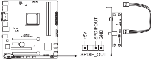
Connecteur audio numérique de la F2A55-M LE
