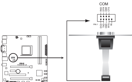
Connecteur COM de la F2A55-M LE
