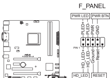
Connecteur système de la F2A55-M LE
