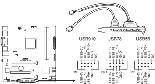
Connecteurs USB 2.0/1.1 de la F2A55-M LE
