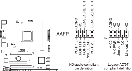
Connecteur pour port audio en façade de la F2A55-M LE
