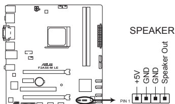
Connecteur pour haut-parleur système de la F2A55-M LE
